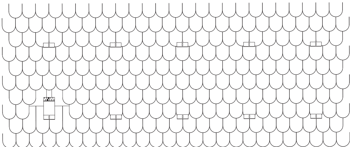
Abb. 3. Bestimmung des Montageortes für tragende Konstruktionsstützen
