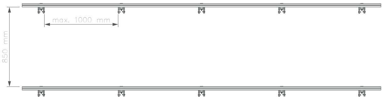
Abb. 2. Anordnung der Montageschienen mit Dachbefestigung
